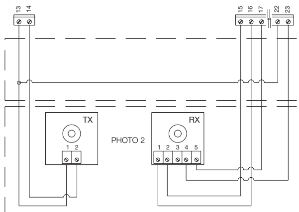
Fig 3C Connexion photo-test avec seulement la photocellule Photo2
